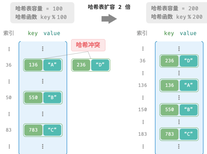
图 6-4 哈希表扩容
