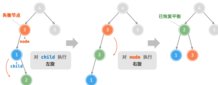
图 7-30 先左旋后右旋
