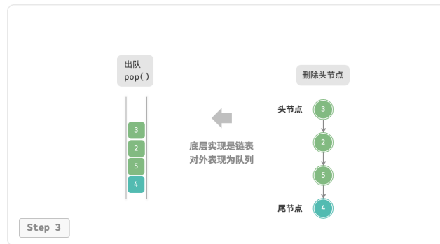
图 5-5 基于链表实现队列的入队出队操作
