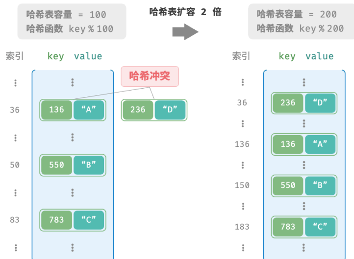
图 6-4 哈希表扩容
