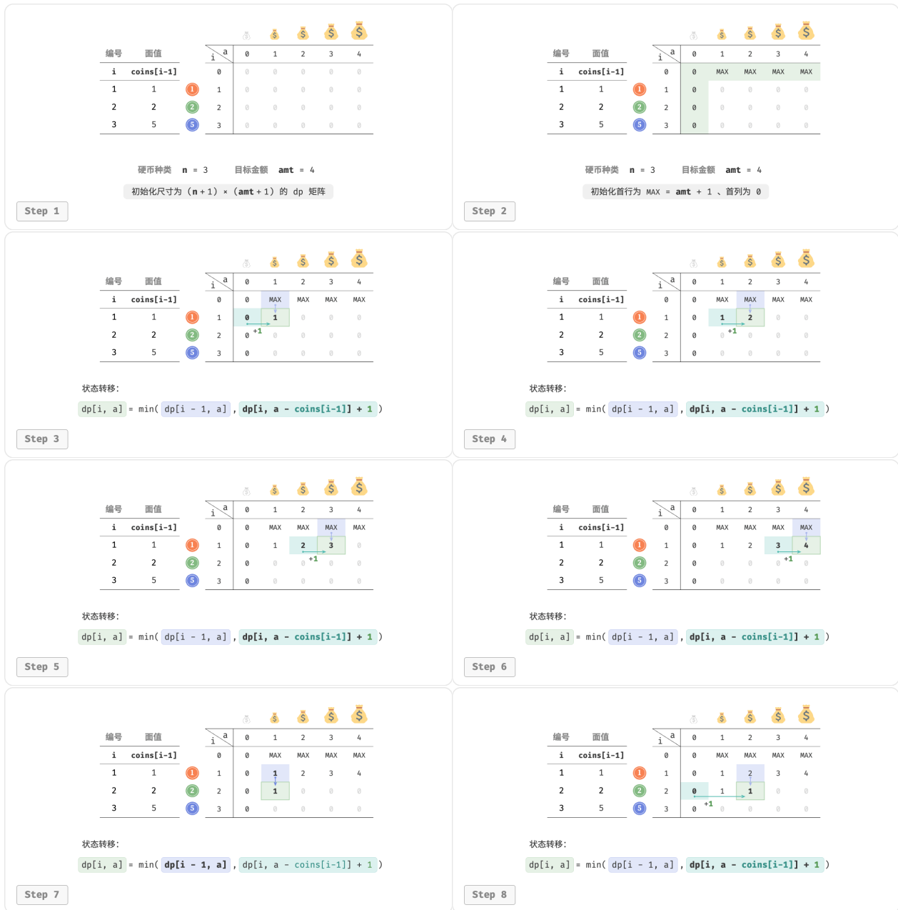
图 14-25 展示了零钱兑换的动态规划过程，和完全背包问题非常相似。
