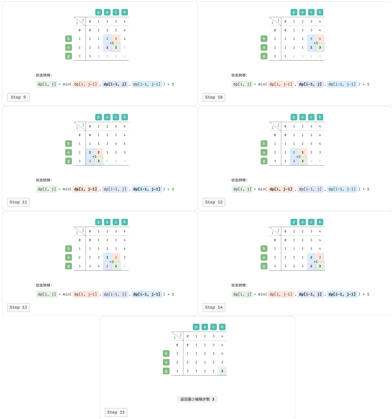
图 14-30 编辑距离的动态规划过程
