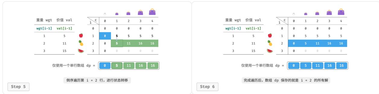
图 14-21 0-1 背包的空间优化后的动态规划过程
